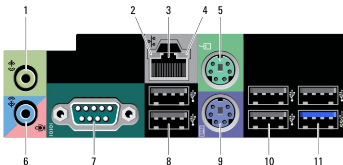
Figura 2. Visão do painel traseiro
