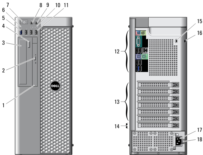
Figura 1. Visão frontal e traseira
